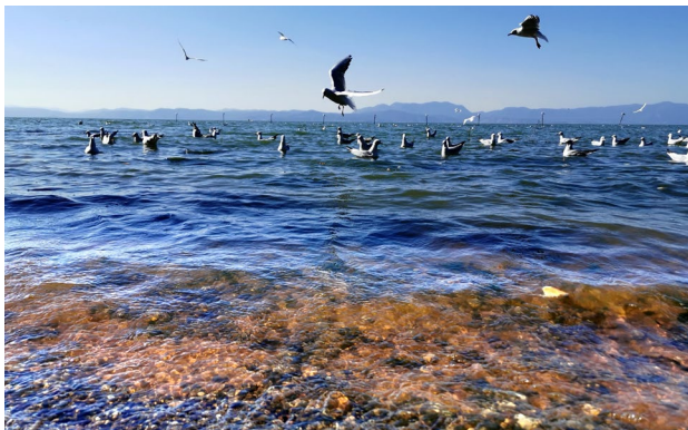
2018年，滇池水质为1988年建立数据监测库30年以来最好水质
